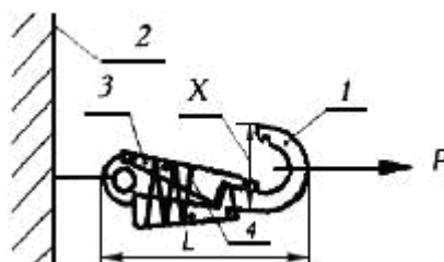
Рисунок 8а - Схема испытания карабина статической нагрузкой
