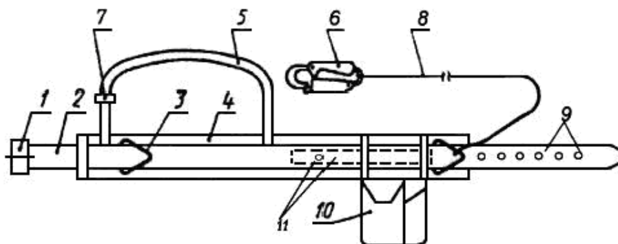
Рисунок 2 - Безлямочный пояс, тип Б (Ба)
