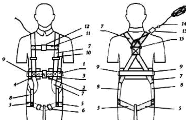
Рисунок 5 - Лямочный пояс, тип Д (Да)
