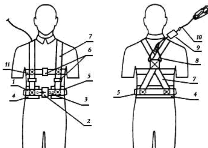
Рисунок 3 - Лямочный пояс, тип В (Ва)
