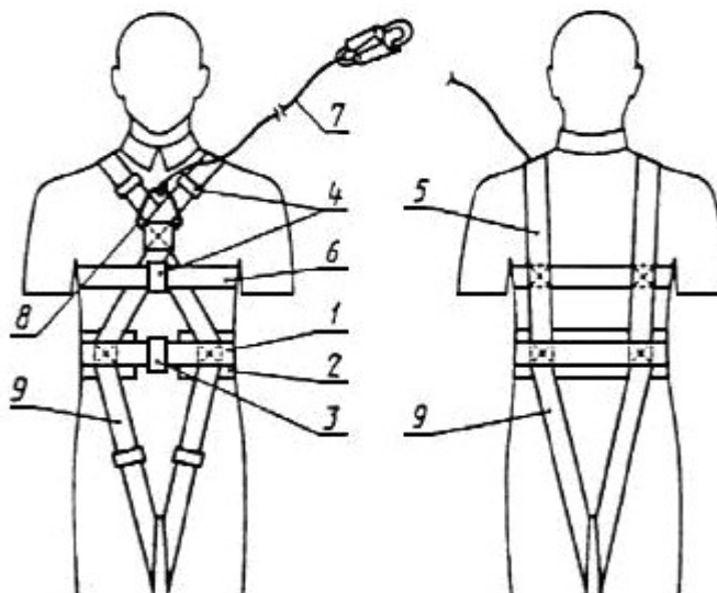
Рисунок 6 - Лямочный пояс, тип Е (Еа)
