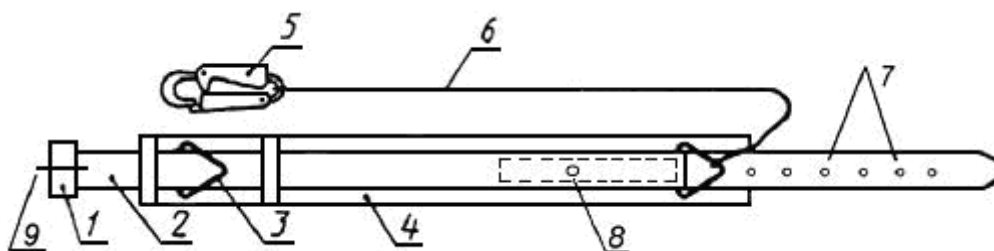
Рисунок 1 - Безлямочный пояс, тип А (Аа)
