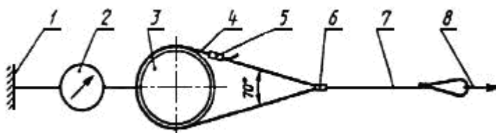
Рисунок 7 - Схема испытания пояса в целом статической нагрузкой
